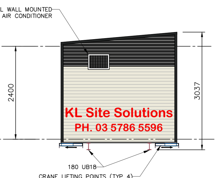
ELEVATION B.
